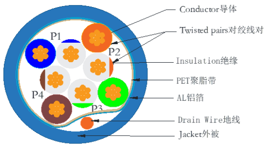
CAT5e F/UTP 4P*26AWG(7/0.16BC,HDPE 0.82mm+PET+AL+D) PVC JACKET OD:5.4
