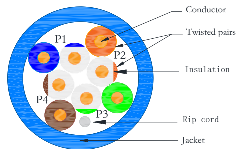
CAT5e U/UTP 4P*24AWG(1/0.5BC, HDPE 0.88mm) PVC JACKET OD:5.2
