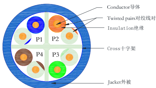
CAT6 U/UTP 4P*23AWG(1/0.57BC,HDPE 1.03mm +CROSS) PVC JACKET OD:6.3
