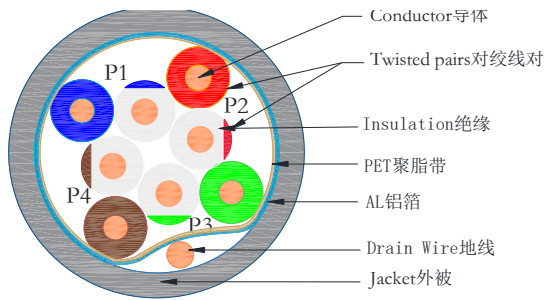
CAT5e F/UTP 4P*24AWG(1/0.5BC,HDPE 1.0mm PET+AL+D) PVC JACKET OD:6.5
