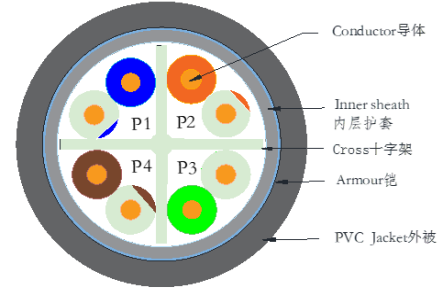
CAT6 U/UTP 4P*23AWG(1/0.57BC,HDPE 1.03mm+CROSS) PVC +A+PVC JACKET OD:9.0
