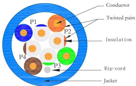
CAT5e U/UTP 4P*24AWG(1/0.5CCA, HDPE 0.88mm) PVC JACKET OD:5.2
