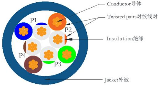
CAT5e UTP 4P*26AWG(7/0.16BC,HDPE 0.77mm) PVC JACKET OD:5.2
