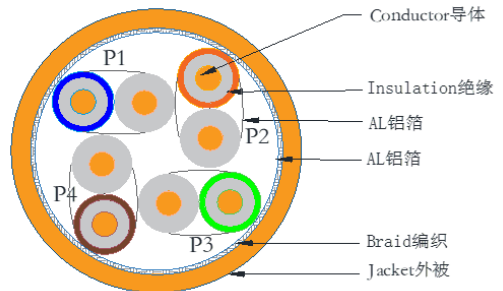
CAT8 SF/FTP 4P*23AWG(1/0.58BC,FM-PE 1.42mm+AL +AL+B) LSZH JACKET OD:8.0
