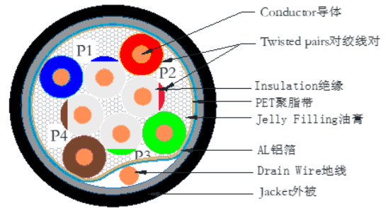
CAT5e F/UTP 4P*24AWG(1/0.5BC,HDPE 1.0mm JELLY+PET+AL+D) PVC+PE JACKET OD:7.4
