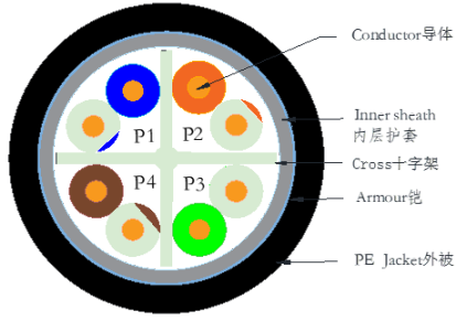
CAT6 U/UTP 4P*23AWG(1/0.57BC,HDPE 1.03mm+CROSS) PVC +A+PE JACKET OD:9.0
